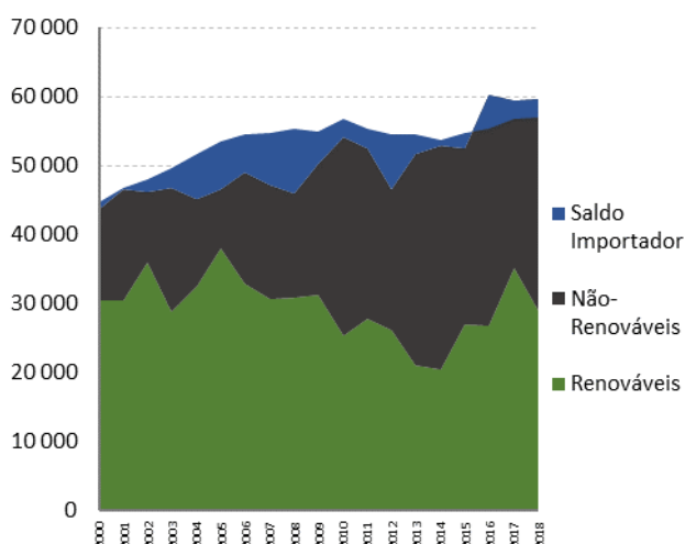
Figura 46 - Evolução da Produção Bruta de Eletricidade e do Saldo Importador em Portugal (GWh) [Fonte: DGE]
