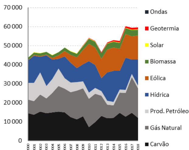
Figura 47 - Evolução da Produção Bruta de Eletricidade em Portugal (GWh) [Fonte: DGE]
