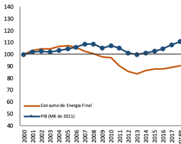
Figura 37 – Evolução do Consumo de Energia Final e do PIB em Portugal (2000 = 100) [Fonte: DGEG, INE]
