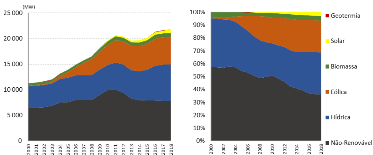
Figura 48 - Evolução da capacidade instalada para a produção de eletricidade em Portugal por tipo de fonte (MW) [Fonte: DGE]
