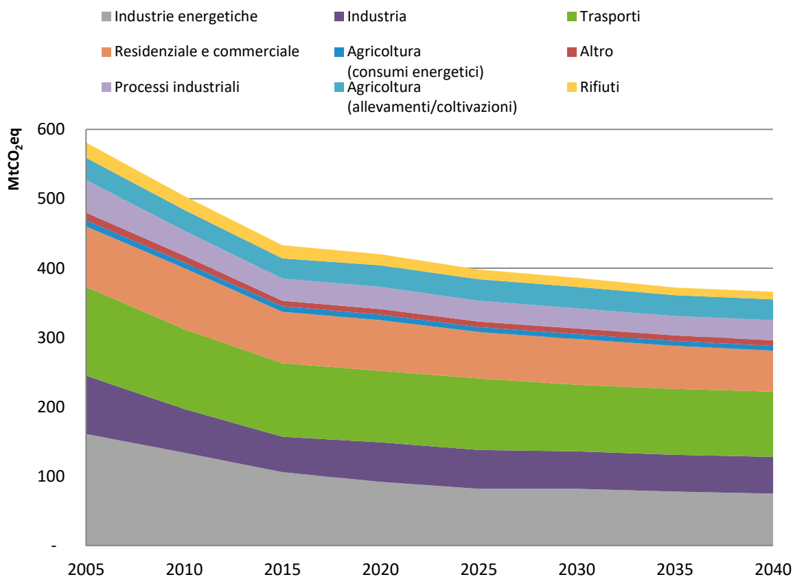
Figura 42 - Emissioni di gas serra (storiche fino al 2015) e secondo lo scenario a politiche correnti disaggregate per settore (MtCO 2 eq) [Fonte: ISPRA]
