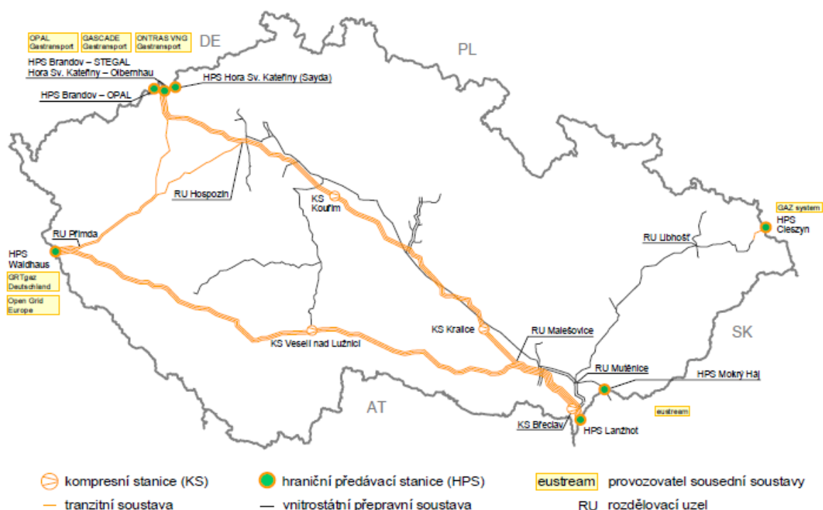
Obrázek č. 11: Přepravní soustava České republiky
