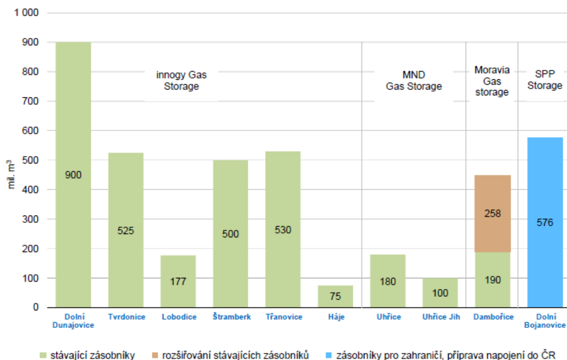
Graf č. 94: Zásobníky plynu – současný stav a rozvoj
