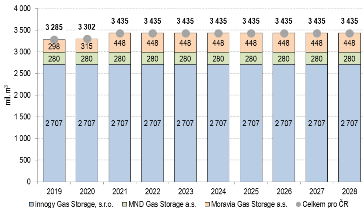
Graf č. 95: Maximální množství uskladněného plynu v letech 2019 až 2028 pro ČR
