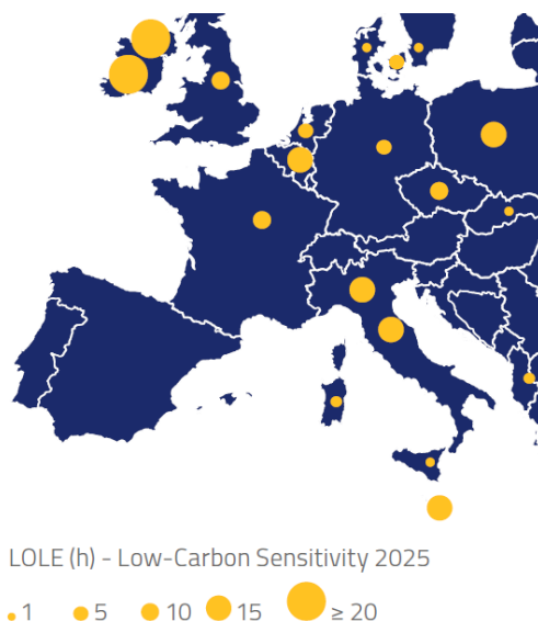
Obrázek č. 7: Výsledky MAF 2018 – scénář Low-Carbon Sensitivity, hodnoty LOLE v roce 2025
