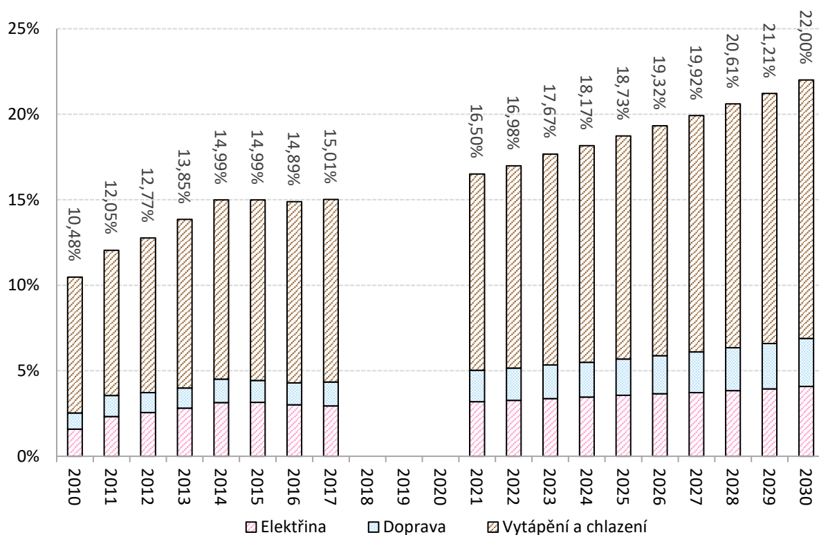
Graf č. 61: Odhad vývoje podílu OZE do roku 2030 v dělení na jednotlivé sektory
