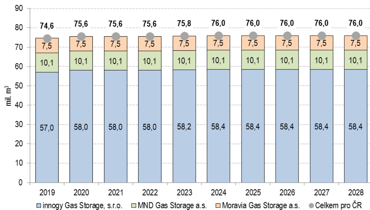
Graf č. 96: Maximální denní výkon těžby plynu v letech 2019 až 2028 pro ČR
