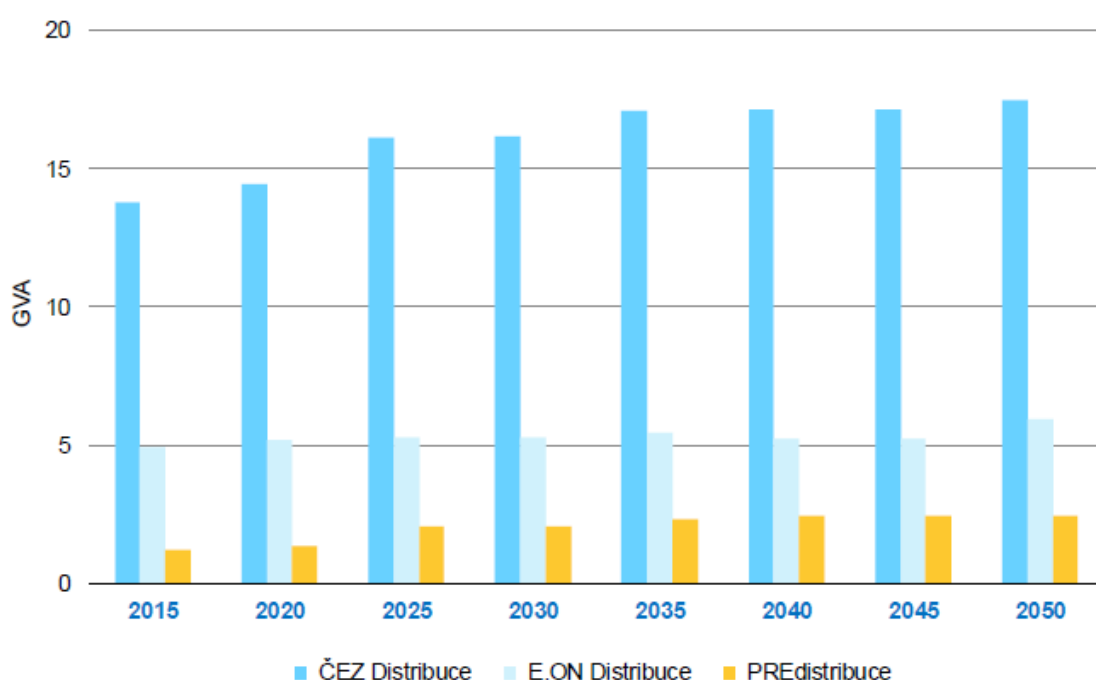
Graf č. 93: Instalovaný výkon transformátorů PS/110 kV (v GVA)
