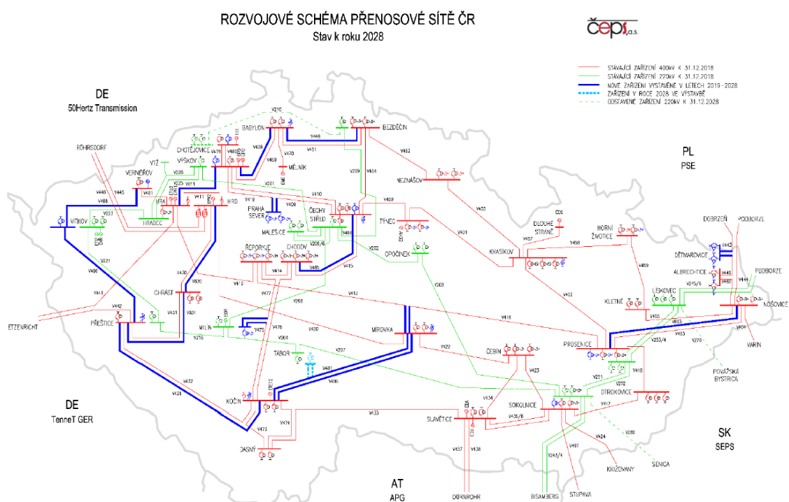
Obrázek č. 13: Rozvojové schéma přenosové sítě ČR (stav k roku 2028)
