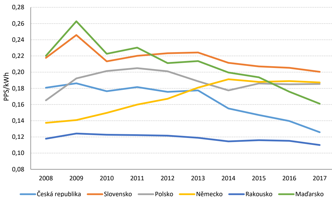
Graf č. 110: Srovnání cen elektřiny mimo domácnosti (pásmo roční spotřeby 500 – 2000 MWh)
