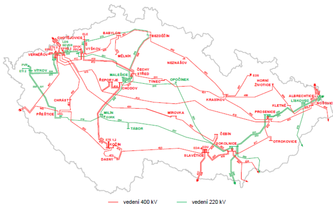
Obrázek č. 10: Přenosová soustava – stávající stav
